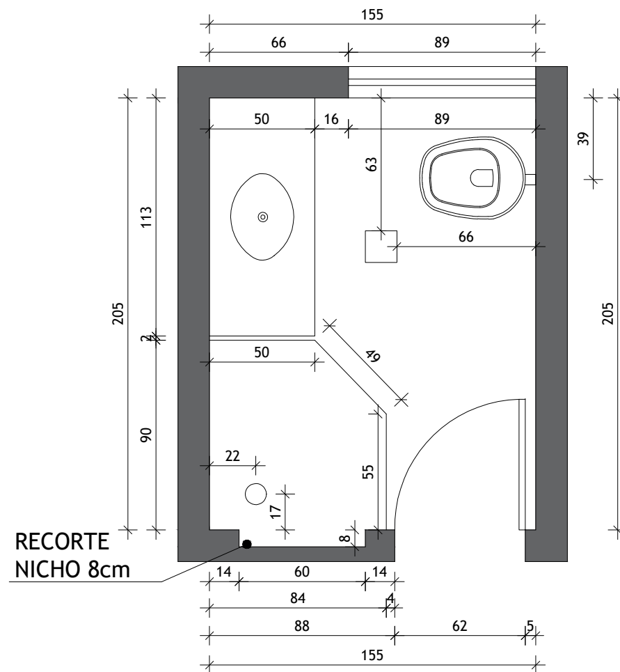
PLANTA DE COTAS ESCALA 1/25
