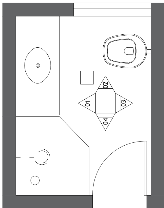
PLANTA DE LAYOUT ESCALA 1/25
