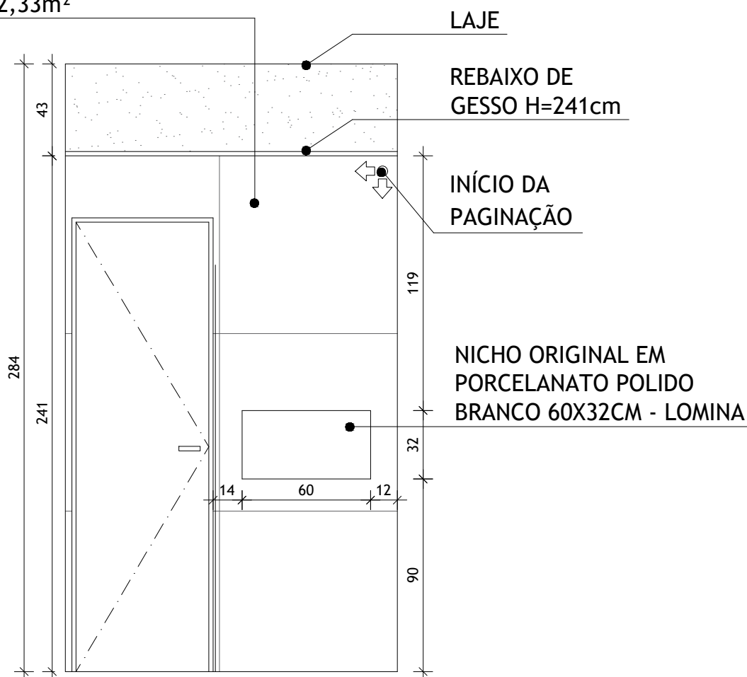
VISTA 4 ESCALA 1/25
