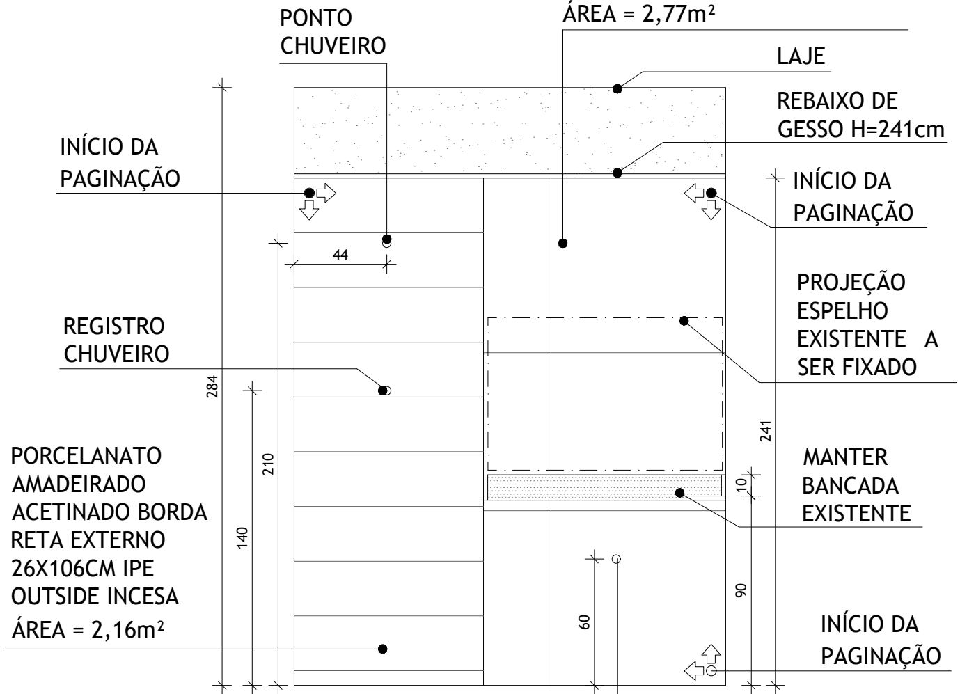
VISTA 1 ESCALA 1/25
