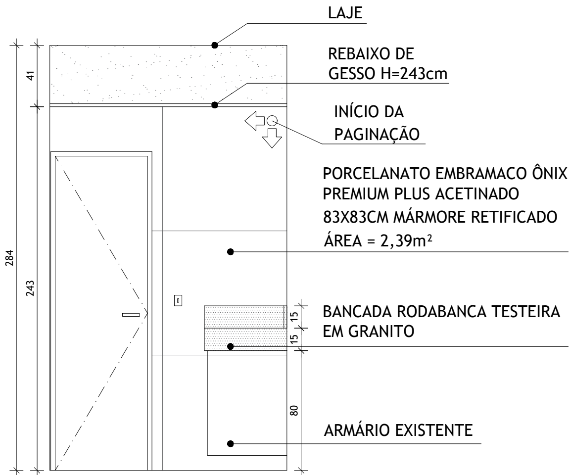
VISTA 3 ESCALA 1/25
