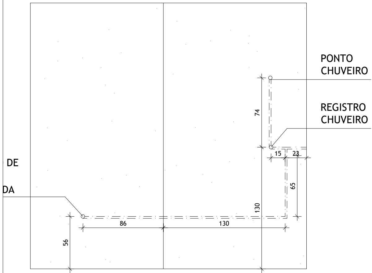
VISTA 1 HIDRÁULICA ESCALA 1/25
