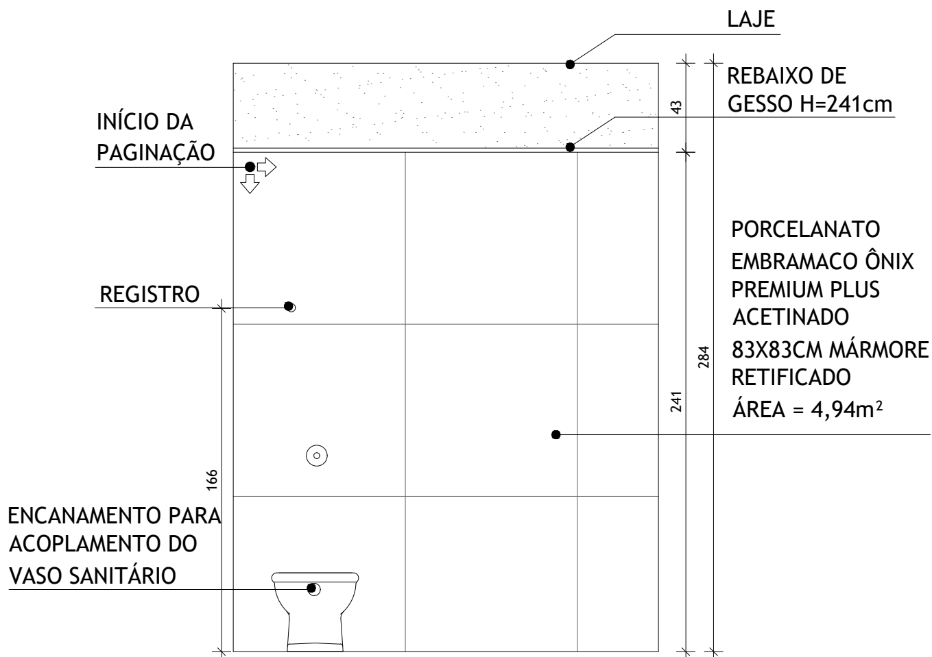
VISTA 3 ESCALA 1/25
