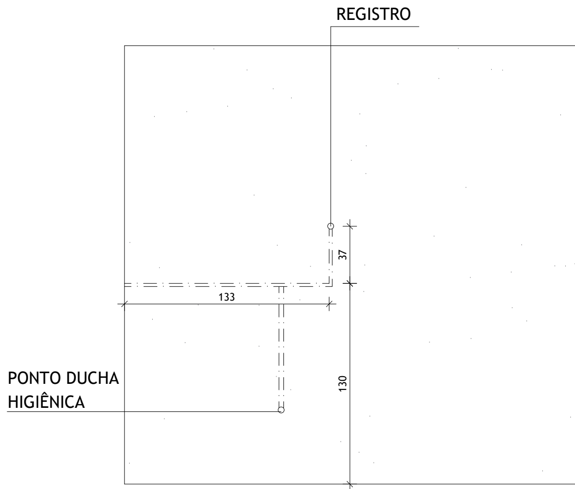
VISTA 4 HIDRÁULICA ESCALA 1/25
