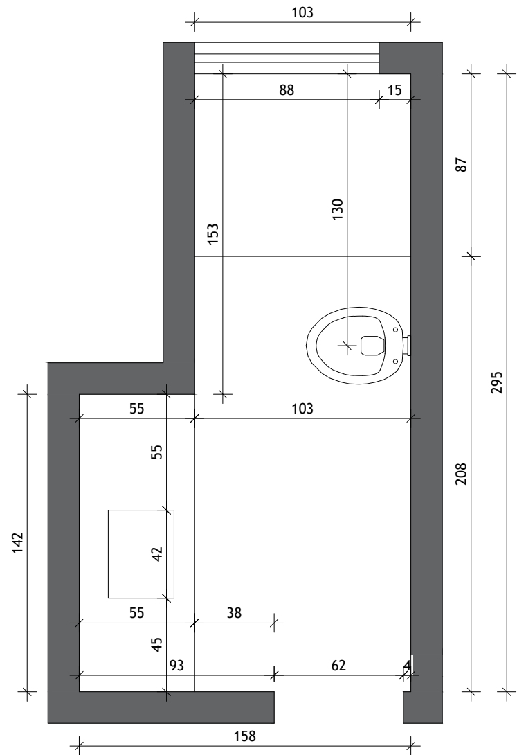
PLANTA DE COTAS ESCALA 1/25
